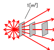
図 7. 照度の定義
